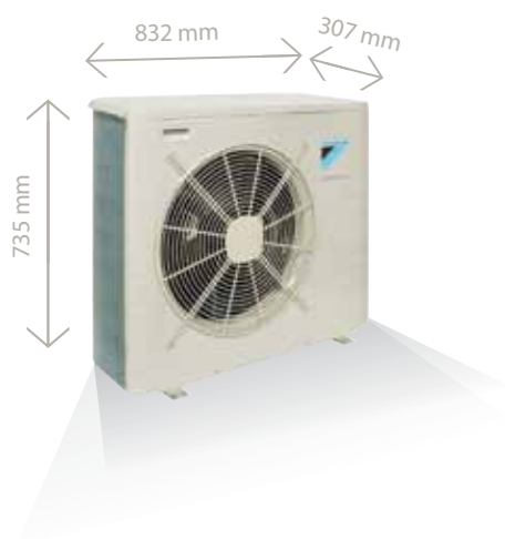
Hőszivattyú kültéri egység
